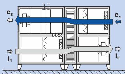
větrání s rekuperačí s dohřevem (s chlazením)
