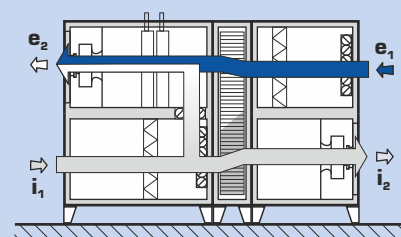
kombinovaný režim (větrání s cirkulací)
